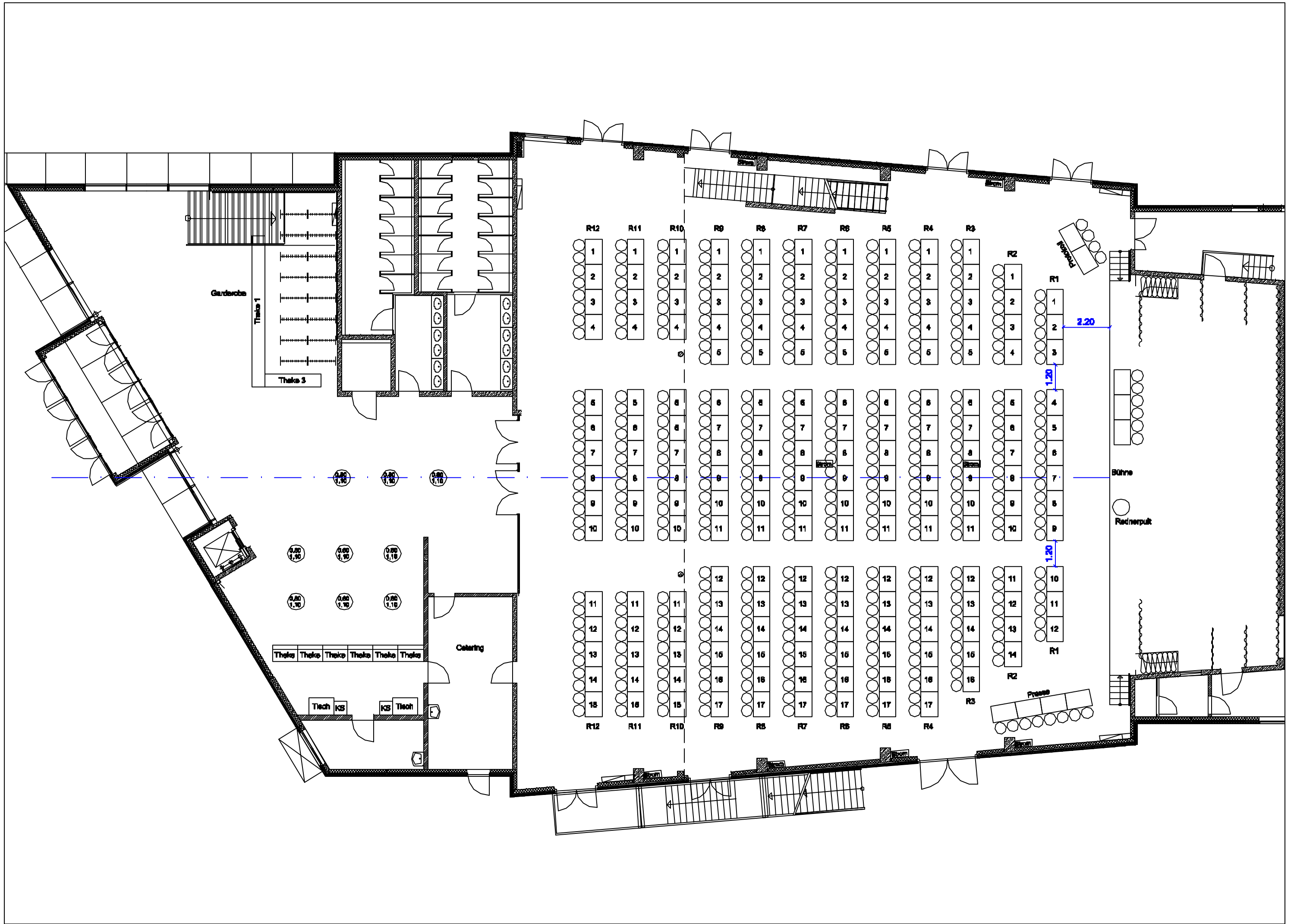
Stadthalle OHZ - Parlamentarische Bestuhlung - EG = 378 Plätze
